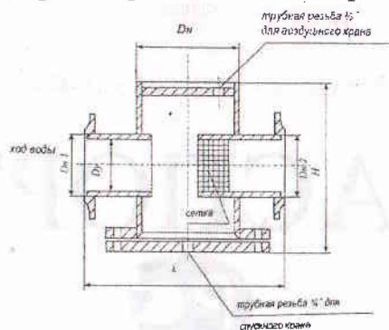
Фланцевое исполнение
